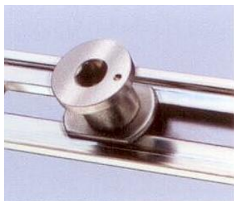
In jedem Bongers Fenster sind umlaufend im Flügel Sicherheitsbauteile mit Pilzzapfen
